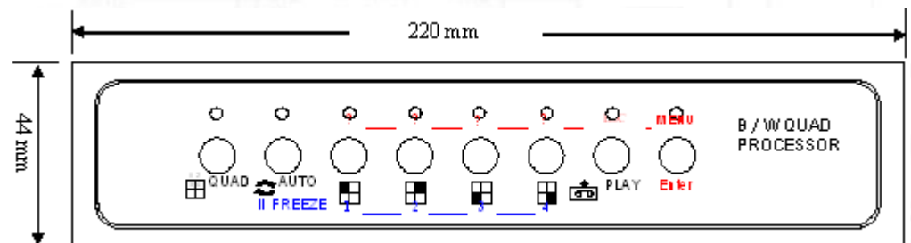
PANELLO FRONTALE
