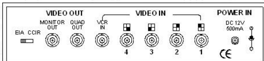
PANELLO POSTERIORE
